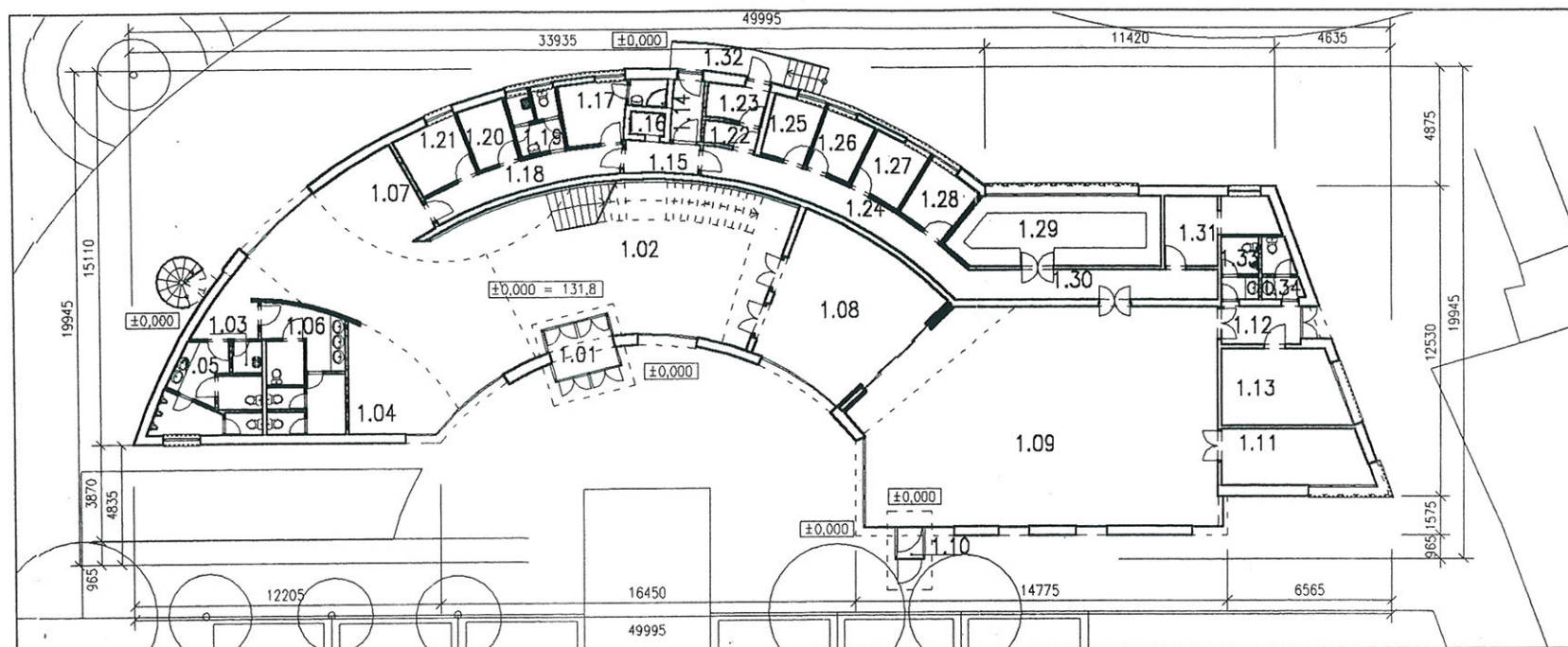
PÔDORYS 1. NP
